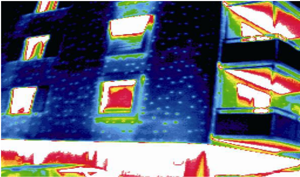
Puentes térmicos en fachada Lana de Roca
